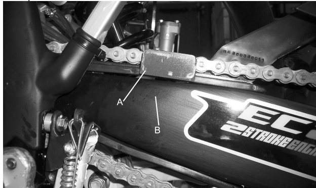
(A). Patín guía cadena. (B). Brazo basculante.
