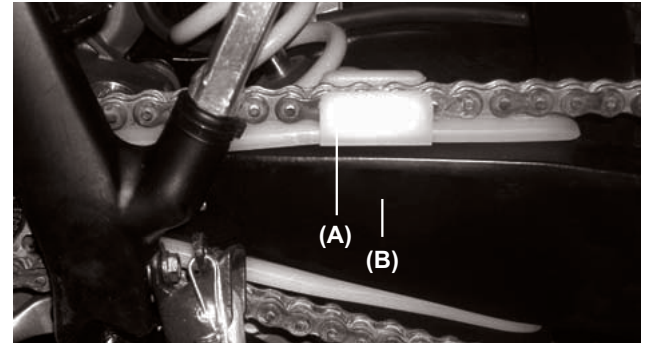
(A). Patín guía cadena. (B). Brazo basculante.
