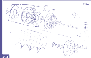
Embrague / Clutch GASGAS EC 2003
