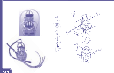
Carburador / Carburetor GASGAS EC 2003
