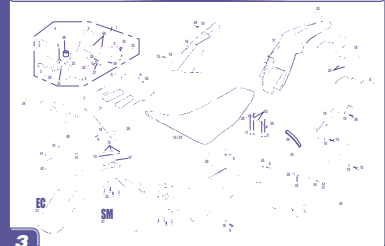
Plásticos / Plastics GASGAS EC 2003
