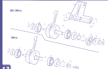
Cigüeñal / Crankshaft GASGAS EC 2003
