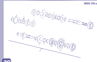
Engranajes cambio / Gear set GASGAS MC 2003
