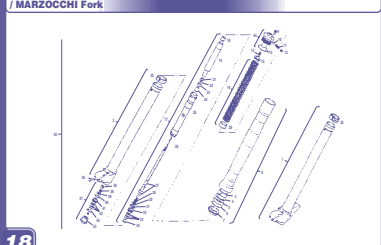
Suspensión MARZOCCHI / MARZOCCHI Fork GASCAS EC 2003
