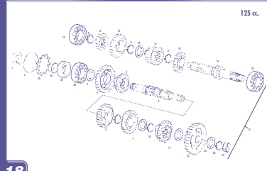
Engranajes cambio / Gear set GASGAS EC 2003
