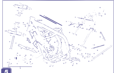
Chasis / Frame GASGAS EC 2003
