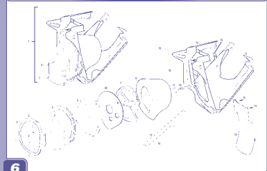
Filtro de aire / Air filter GASGAS EC 2003
