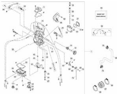
TAV.12 Carburatore - Carburator - Carburateur - Vergaser - Carburador
