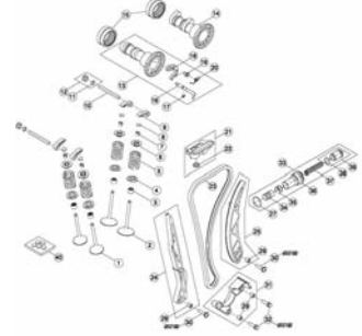
TAV.11A Valvole-Catena distribuzione - Valves-Timing chain - Soupapes-Chaine de distribution - Ventil-Steuerkette - Válvulas-Cadena de distribución
