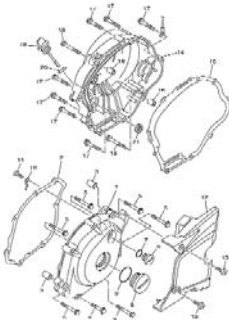
TAV.9 Coperchio frizione - Clutch cover - Couvercle d'embrague - Kupplungsdeckel - Tapa embrague
