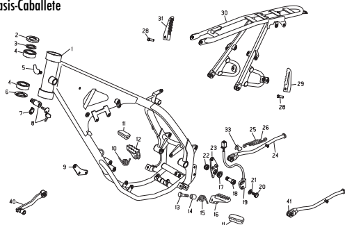
TAV.22 Telaio-Cavalletto - Chassis-Central stand - Châssis-Bequille - Rahmen-Ständer - Chasis-Caballette
