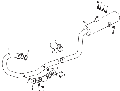
TAV.23 Marmitta - Silencer - Silencieux - Auspufftopf - Silenciador
