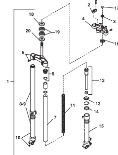
TAV.19A Forcella anteriore - Front fork - Fourche AV. - Vorderradgabel - Horquilla delantera
