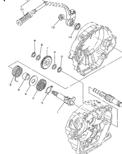
TAV.10 Leva messa in moto - Start. lever - Levier du démarrage - Kickstarterhebel - Palanca de arranque
