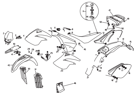
TAV.29 Carenature - Fairings - Carenages - Verkleidungen - Carenados
