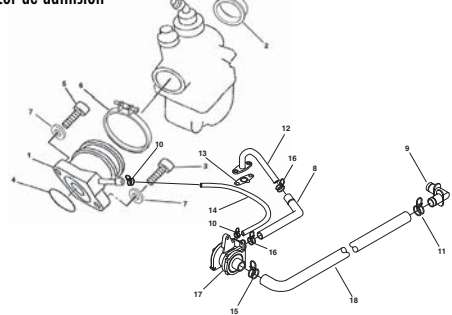
TAV.6 Raccordo d'ammissione - Induction pipe - Raccord d'admission - Ansaugstutzen - Racor de admision
